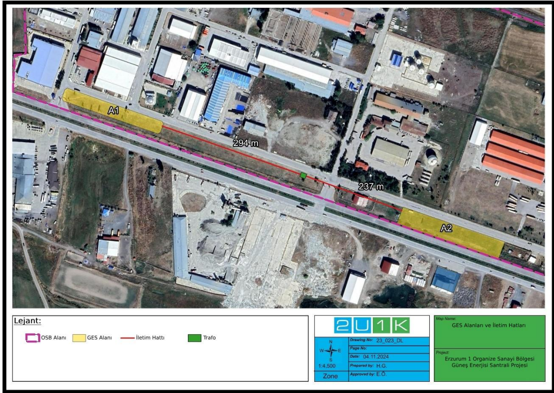
Şekil 2-7. A1 ve A2 Enerji İletim Hattı
