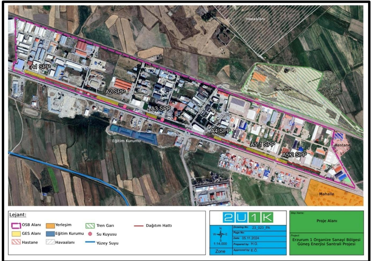
Şekil 2-3. Projenin EOSB Tesisleri İçerisindeki Konumu
